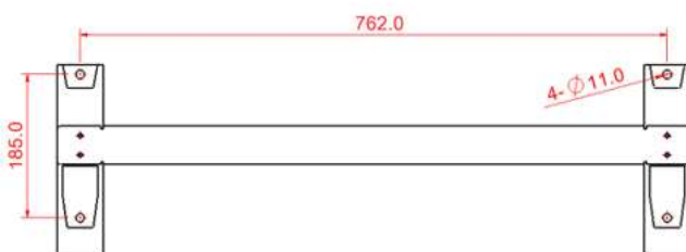
취부홀 치수
